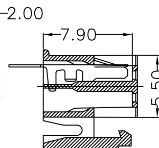
截面 A-A
