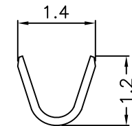
SEC:B-B
