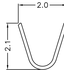
SEC:A-A
