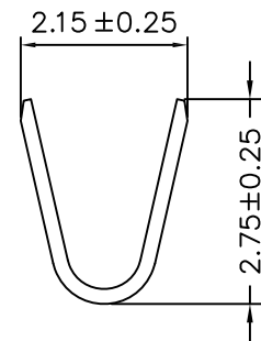
SEC:A-A
