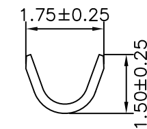
SEC:B-B
